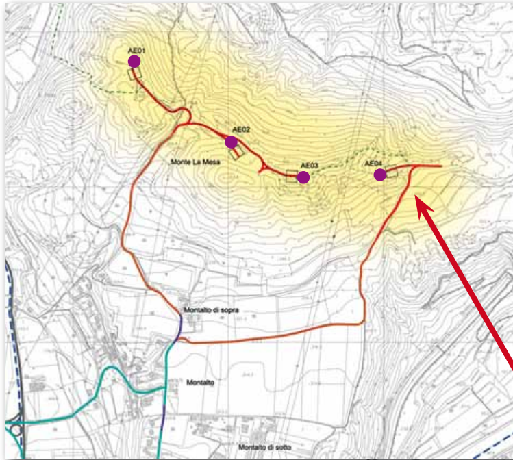
Parco aerogeneratori
